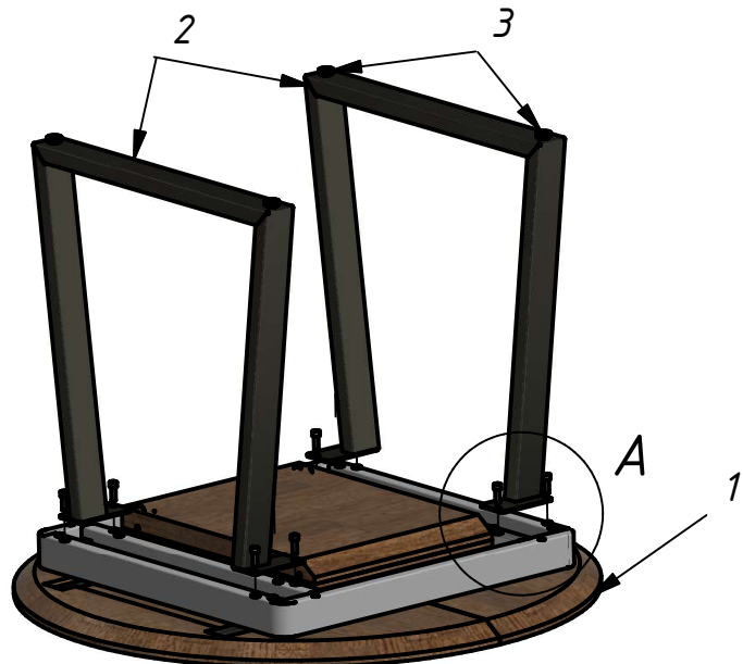
Схема сборки ножки TrP - 80, TrP - 60 к раме с механизмом "бабочка" Раунд, Вейв.
