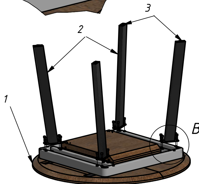
Схема сборки ножки ЕЖ/Р - 80 к раме с механизмом "бабочка" Раунд, Вейв.
